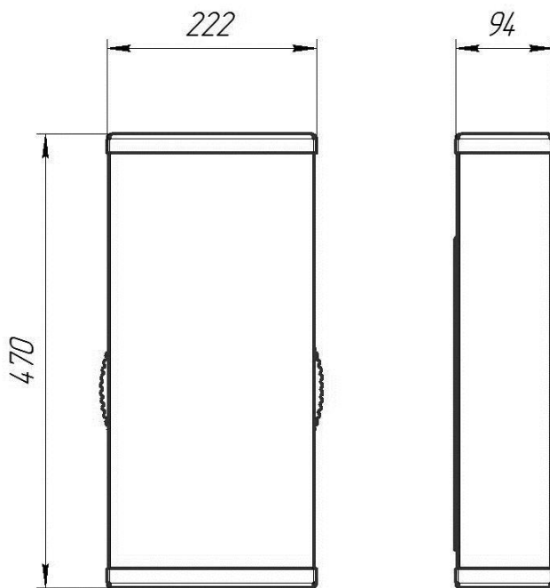
Габаритные размеры шумоглушителя
