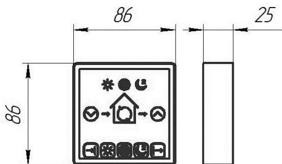
Габаритные размеры контроллера
